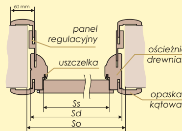
drzwi z ościeżnicą Regulowaną Model 2000
