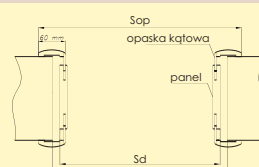
Tunel ZT z opaskami OK7
