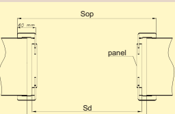
Tunel ZN z opaskami OK6
