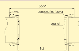
Tunel ZT z opaskami OK4
