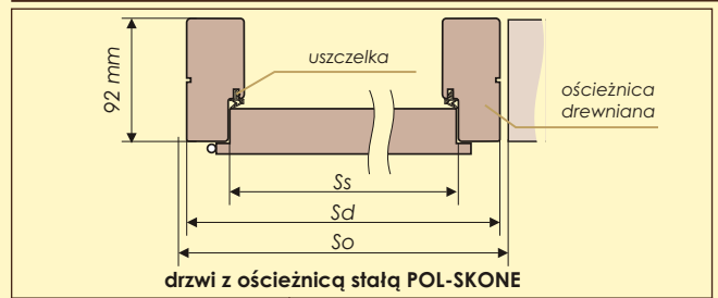
drzwi z ościeżnicą stałą POL-SKONE
