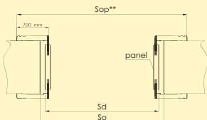
Tunel ZX/ZY z opaskami OK9
