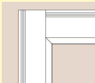
WZÓR A (100 mm) (w ościeżnicach NOBLE)
