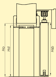
drzwi przesuwne – system naścienny z zabudową tunelową ZN OK6
