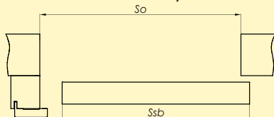
drzwi przesuwne – system naścienny bez zabudowy
