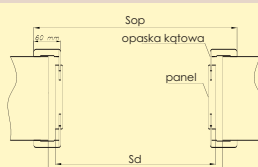
Tunel ZT z opaskami OK6
