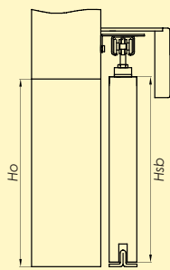
drzwi przesuwne – system naścienny bez zabudowy
