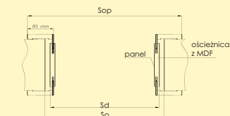
Tunel ZX/ZY z opaskami OK8
