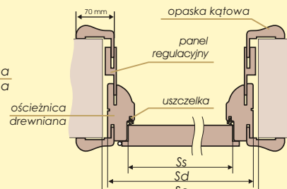
drzwi z ościeżnicą Regulowaną Model RETRO
