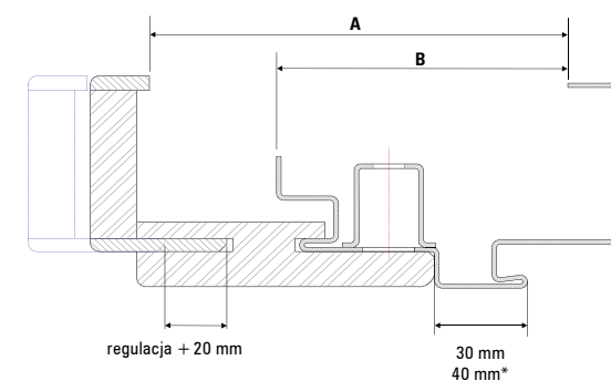
Rysunek (poglądowy) przekroju ościeżnicy PROJEKT
