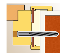
Montaż na piankę i kotwy w ścianie murowanej
