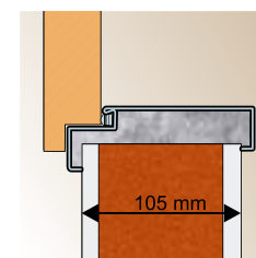
Ościeżnica kątowa duża – na murze o grubości 100 mm
