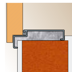
Ościeżnica kątowa duża – na murze o grubości powyżej 100 mm
