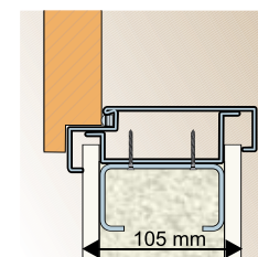
Ościeżnica kątowa duża – na ścianach gipsowo-kartonowych
