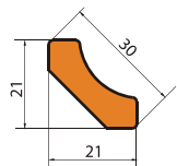
ĆWIERĆWAŁEK WKŁĘŚŁY
